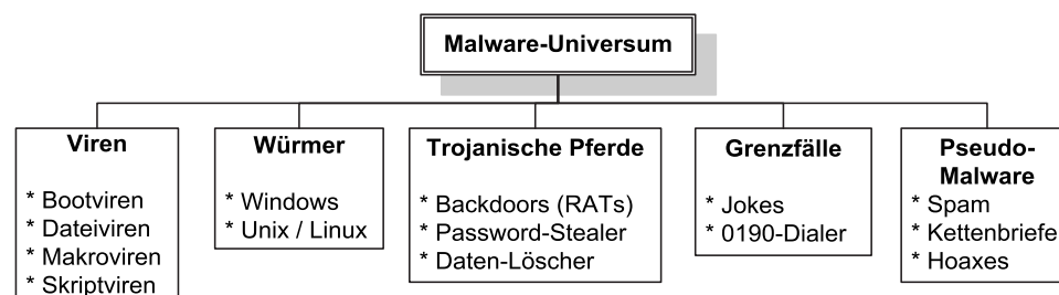
Bild 1 Klassifizierung von Malware-Arten
